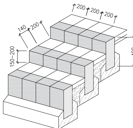
LA LINIA – Multablok 20/40/14 pískovaný ze dvou stran
