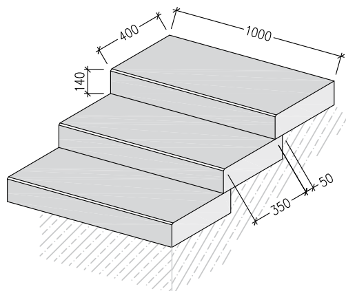
LA LINIA – schod 40/100/14 pískovaný ze čtyř stran
