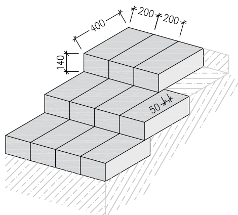
LA LINIA – Multablok 20/40/14 pískovaný ze dvou stran
